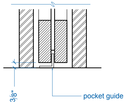
Pocket Door
