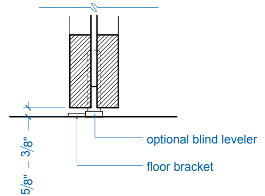
Fixed Door
