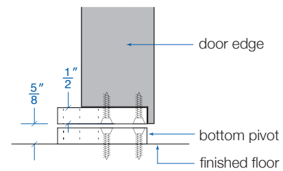
(PVO) Pivoting Offset
